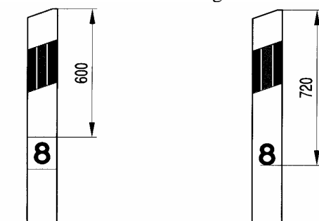
Rys. 11.2.2. Umieszczenie znaku hektometrowego U-6 na słupku prowadzącym U-1
