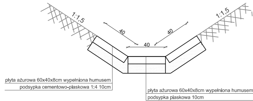
SZCZEGÓŁ "A" Umocnienie dna rowu przy pochyleniu podłużnym powyżej 3%
