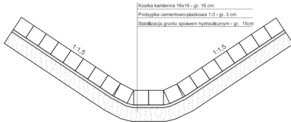
SZCZEGÓŁ "B" Umocnienie rowu przy przepustach
