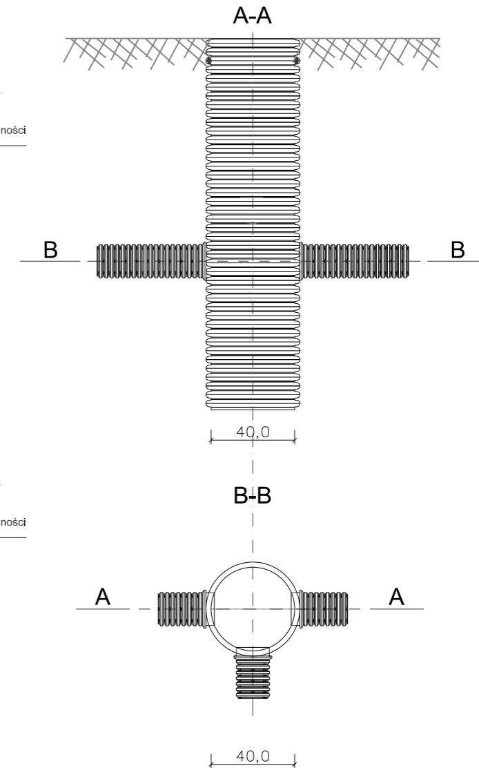
SZCZEGÓŁ "F" Studnia drenarska DN400
