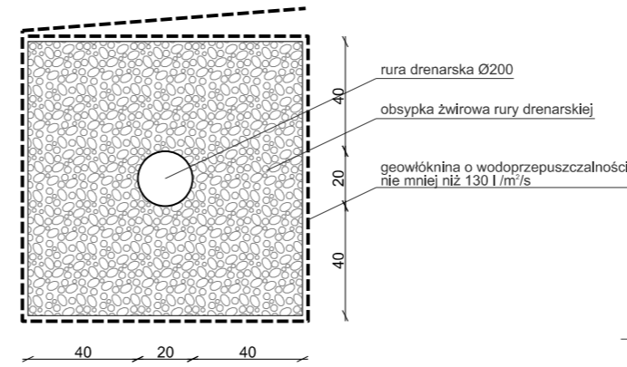
SZCZEGÓŁ "D" Obsypka rury drenarskiej Ø315
