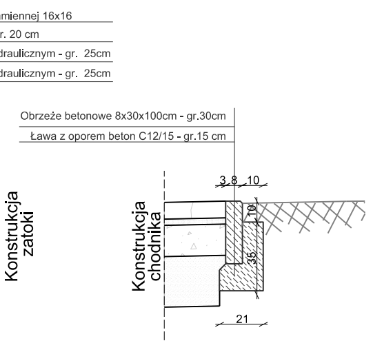
SZCZEGÓŁ "F" Ułożenie obrzeża
