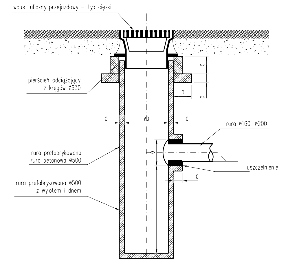
SZCZEGÓŁ "G" Wpust uliczny bezsyfonowy
