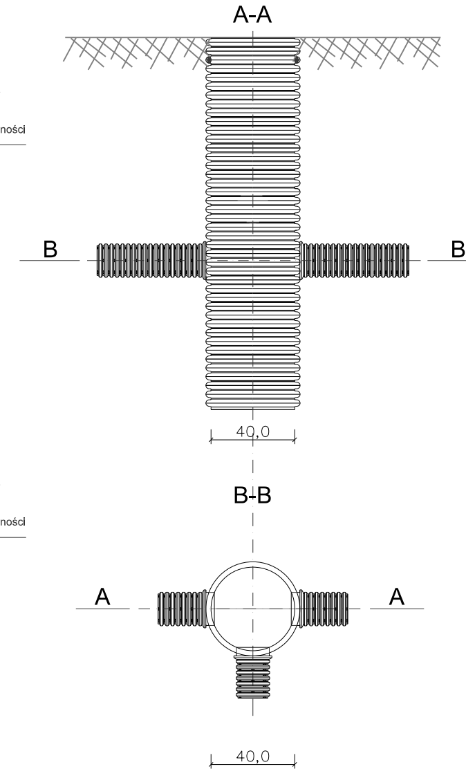
SZCZEGÓŁ "F" Studnia drenarska DN400
