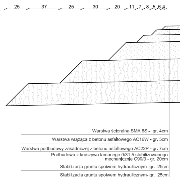
SZCZEGÓŁ "G" Schodkowanie konstrukcji nawierzchni nowa konstrukcja nawierzchni KR3
