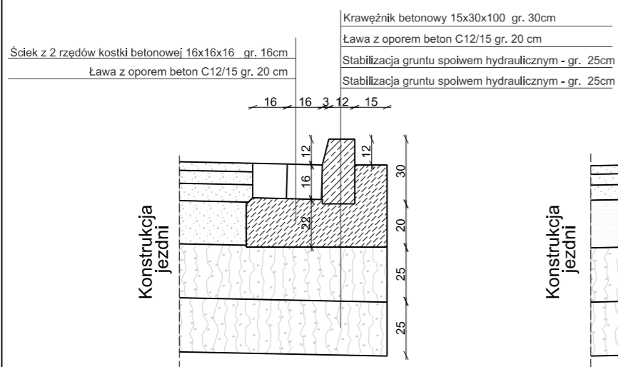
SZCZEGÓŁ "A" Ułożenie krawężnika wyniesionego ze ściekiem z kostki
