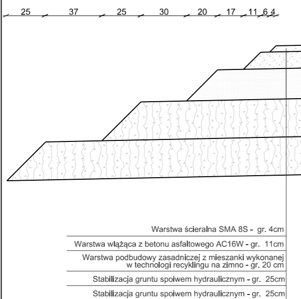
SZCZEGÓŁ "F" Schodkowanie konstrukcji nawierzchni nawierzchnia z recyklingiem KR3
