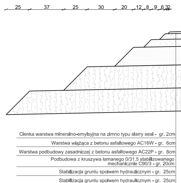
SZCZEGÓŁ "H" Schodkowanie konstrukcji nawierzchni cienka warstwa bitumiczna na zimno KR3
