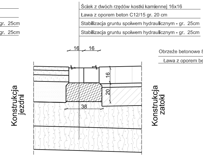
SZCZEGÓŁ "E" Ułożenie ścieku z kostki kamiennej wzdłuż zatoki autobusowej
