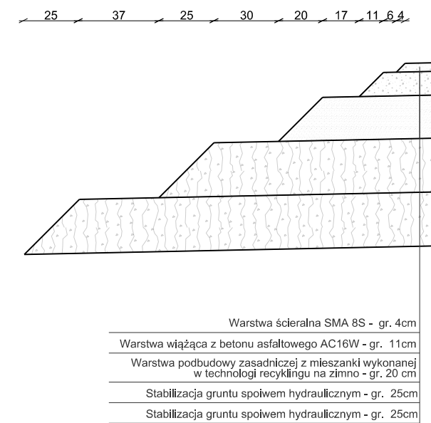
SZCZEGÓŁ "I" Schodkowanie konstrukcji nawierzchni nawierzchnia z recyklingiem KR3
