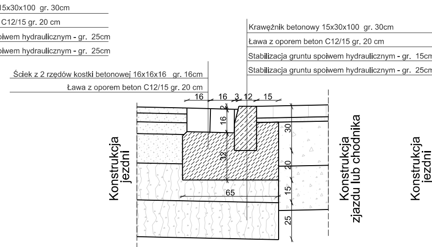
SZCZEGÓŁ "C" Ułożenie krawężnika obniżonego ze ściekiem z kostki
