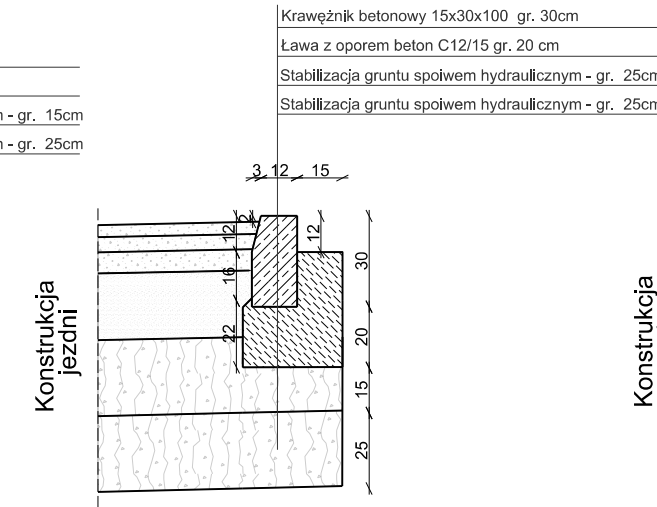
SZCZEGÓŁ "D" Ułożenie krawężnika obniżonego
