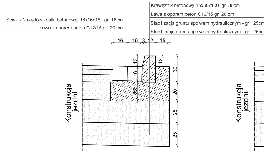
SZCZEGÓŁ "A" Ułożenie krawężnika wyniesionego ze ściekiem z kostki
