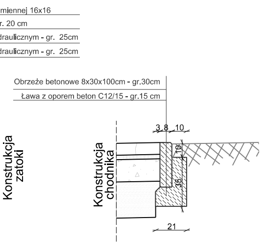
SZCZEGÓŁ "F" Ułożenie obrzeża
