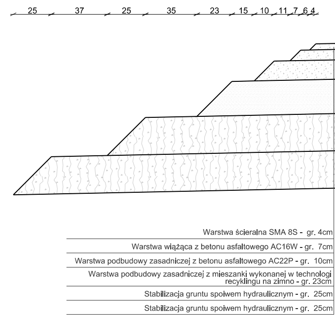
SZCZEGÓŁ "G" Schodkowanie konstrukcji nawierzchni nawierzchnia z recyklingiem KR5
