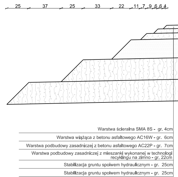
SZCZEGÓŁ "H" Schodkowanie konstrukcji nawierzchni nawierzchnia z recyklingiem KR4
