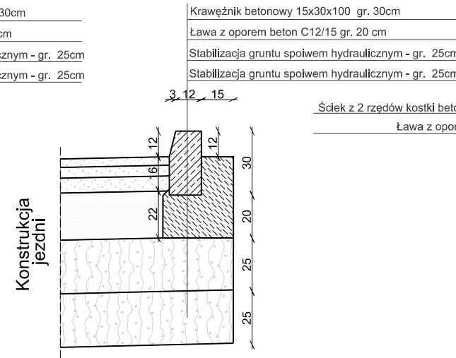
SZCZEGÓŁ "B" Ułożenie krawężnika wyniesionego
