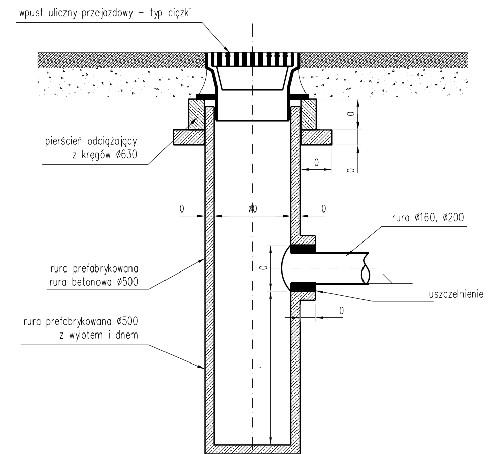
SZCZEGÓŁ "G" Wpust uliczny bezsyfonowy
