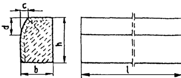
Rys. 1. Wymiarowanie krawężników
